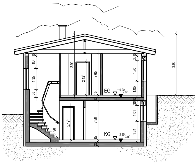
Schnitt A
