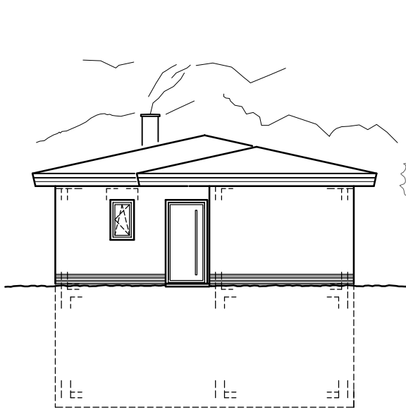
Nordansicht
